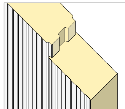
WSJ: giunto speciale a labirinto su richiesta.
